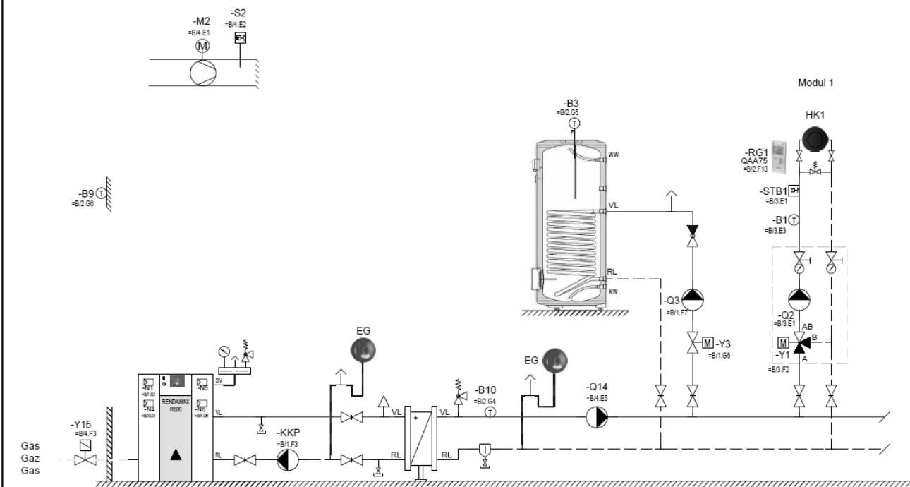
2-5-B-C: 1 отопительный контур и ГВС + пластинчатый теплообменник
