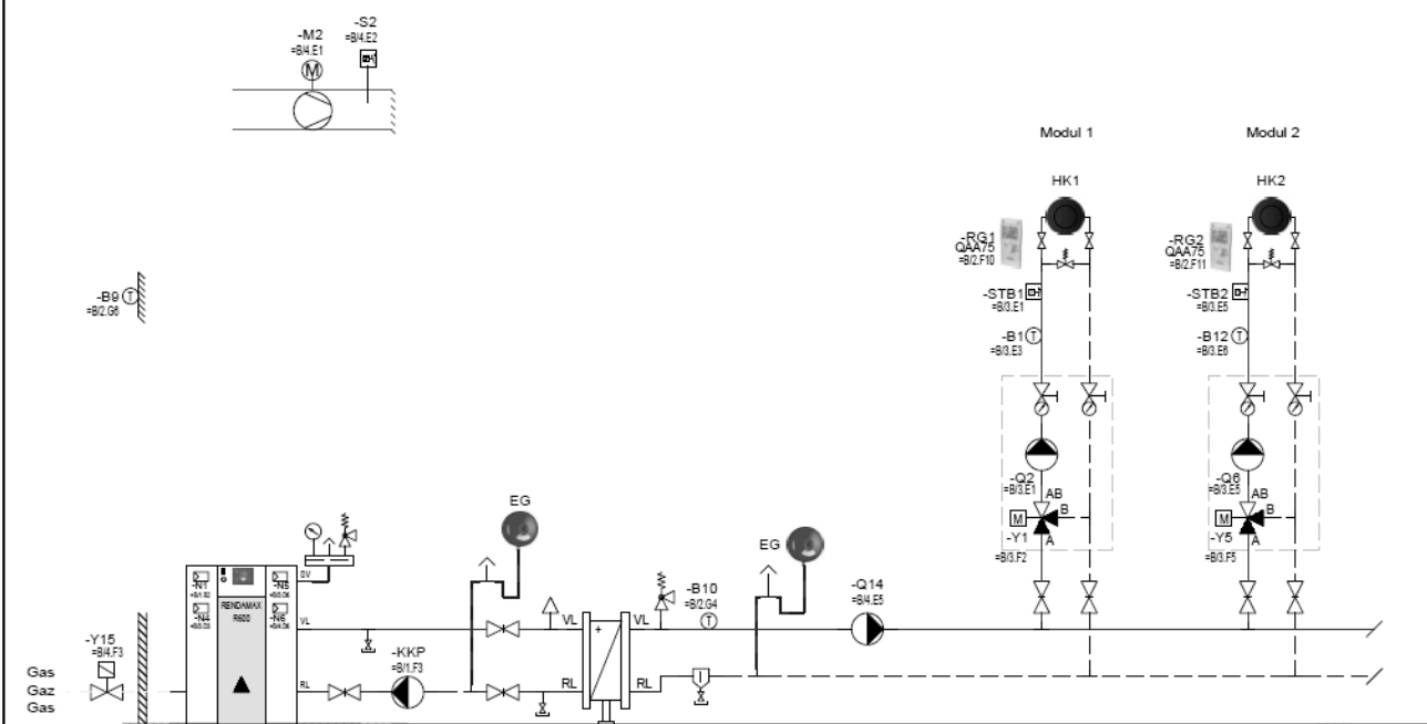
4-B-C: 2 отопительных контура + пластинчатый теплообменник
