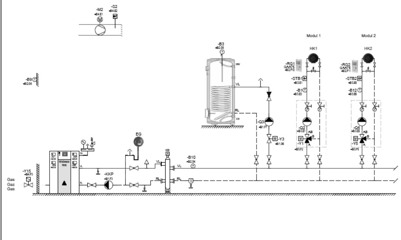
4-5-A-C: 2 отопительных контура и ГВС + гидравлический разделитель
