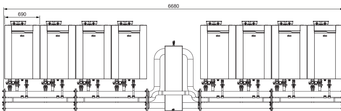
THISION L PLUS — настенный монтаж в ряд 8 котлов
