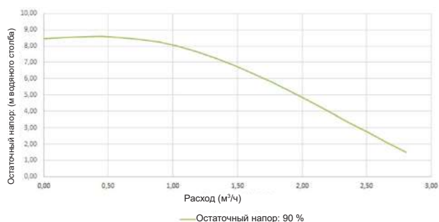
Характеристика насоса, модель котла 60–70
