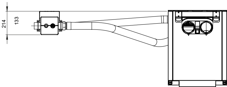
1 котел THISION L PLUS
