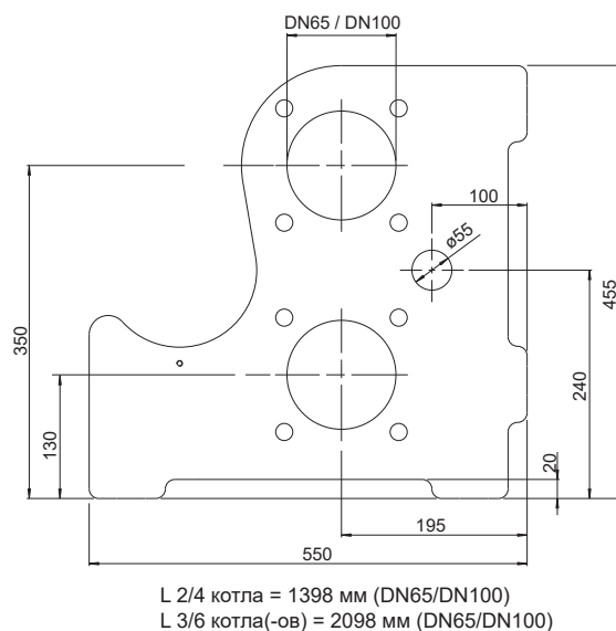
Габаритные размеры главного коллектора
