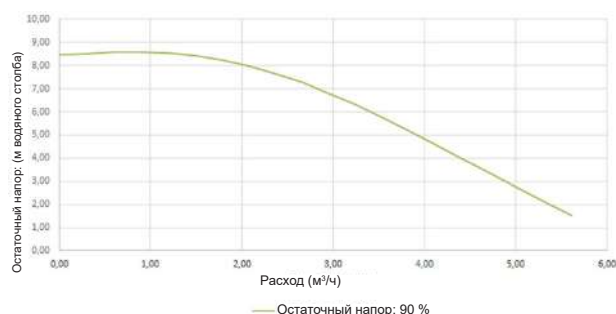
Характеристика насоса, модель котла 120–140
